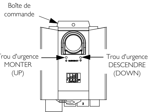
FIGURE 3.2 Déverrouillage d'urgence primaire
